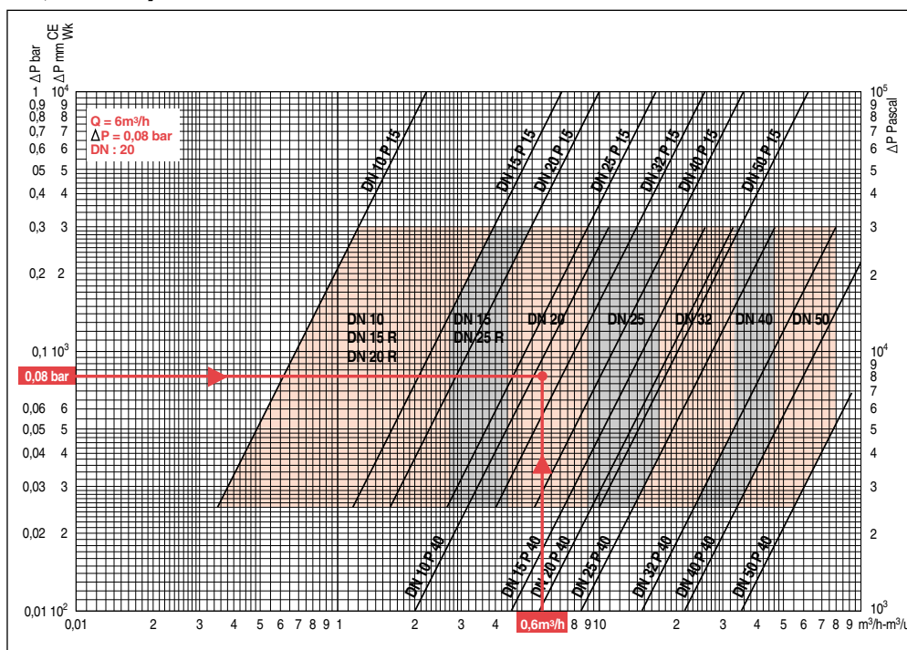
график выбора муфтовых балансировочных клапанов 51, 75 от Ду 10 до 50
